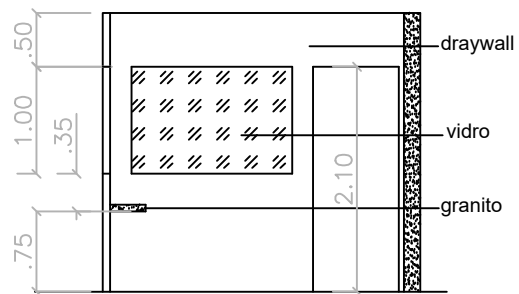
Corte esquemático AA
