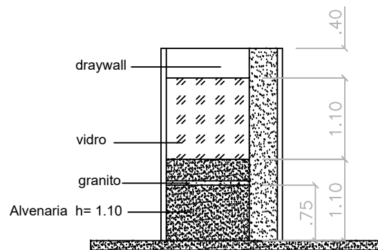
Corte esquemático BB
