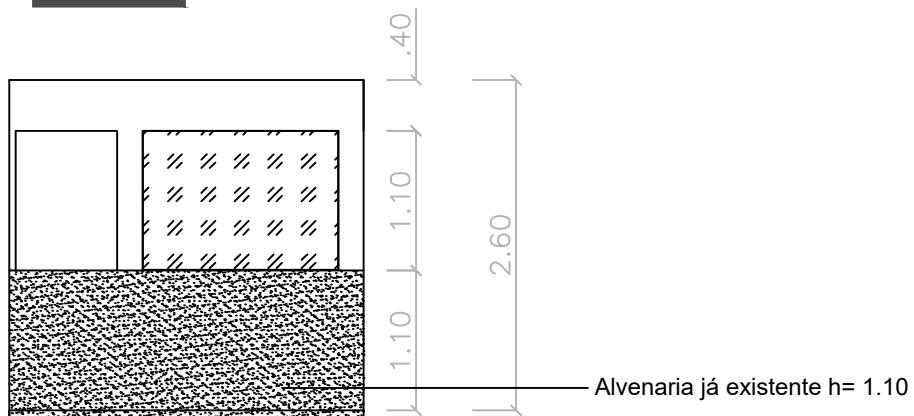
Corte esquemático AA
