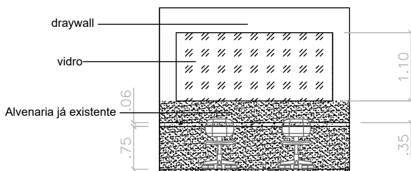
Corte esquemático BB
