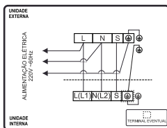
Esquema de ligação das unidades PISO-TETO (PD) e CASSETE (KD) Modelo 18/24/30/36 - 220V ~60Hz - (FRIO)
