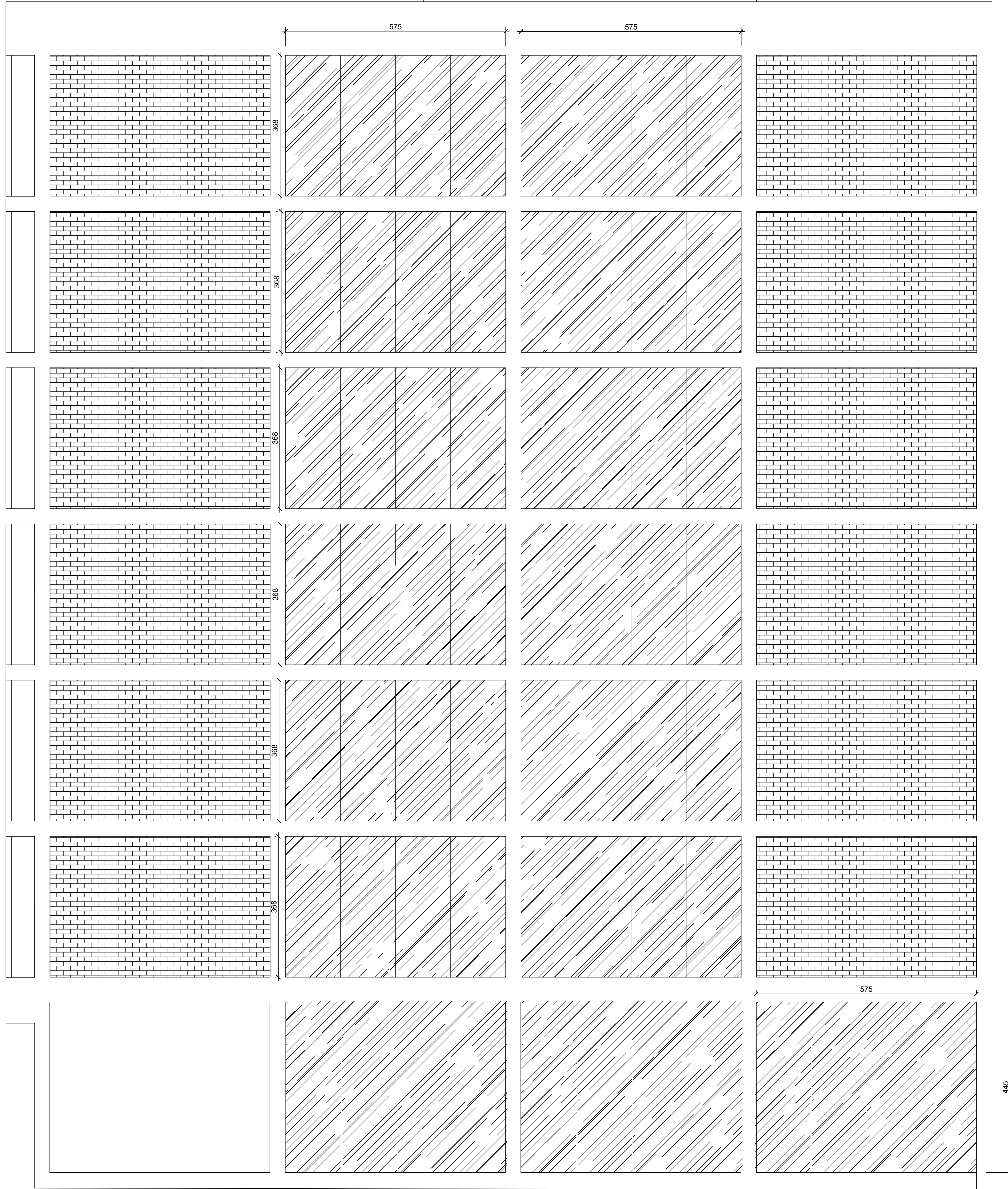
FACHADA LESTE
