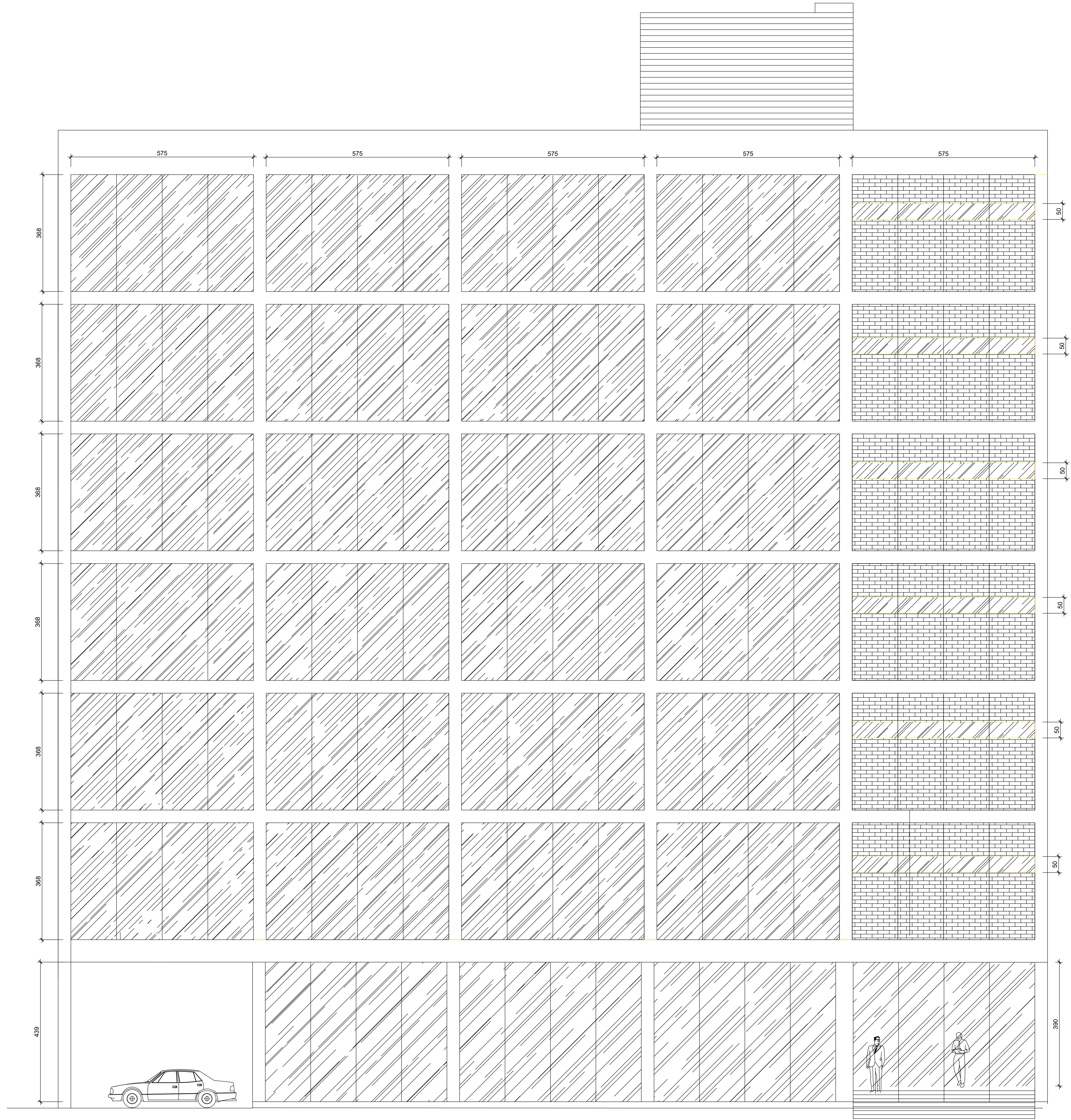
FACHADA NORTE
